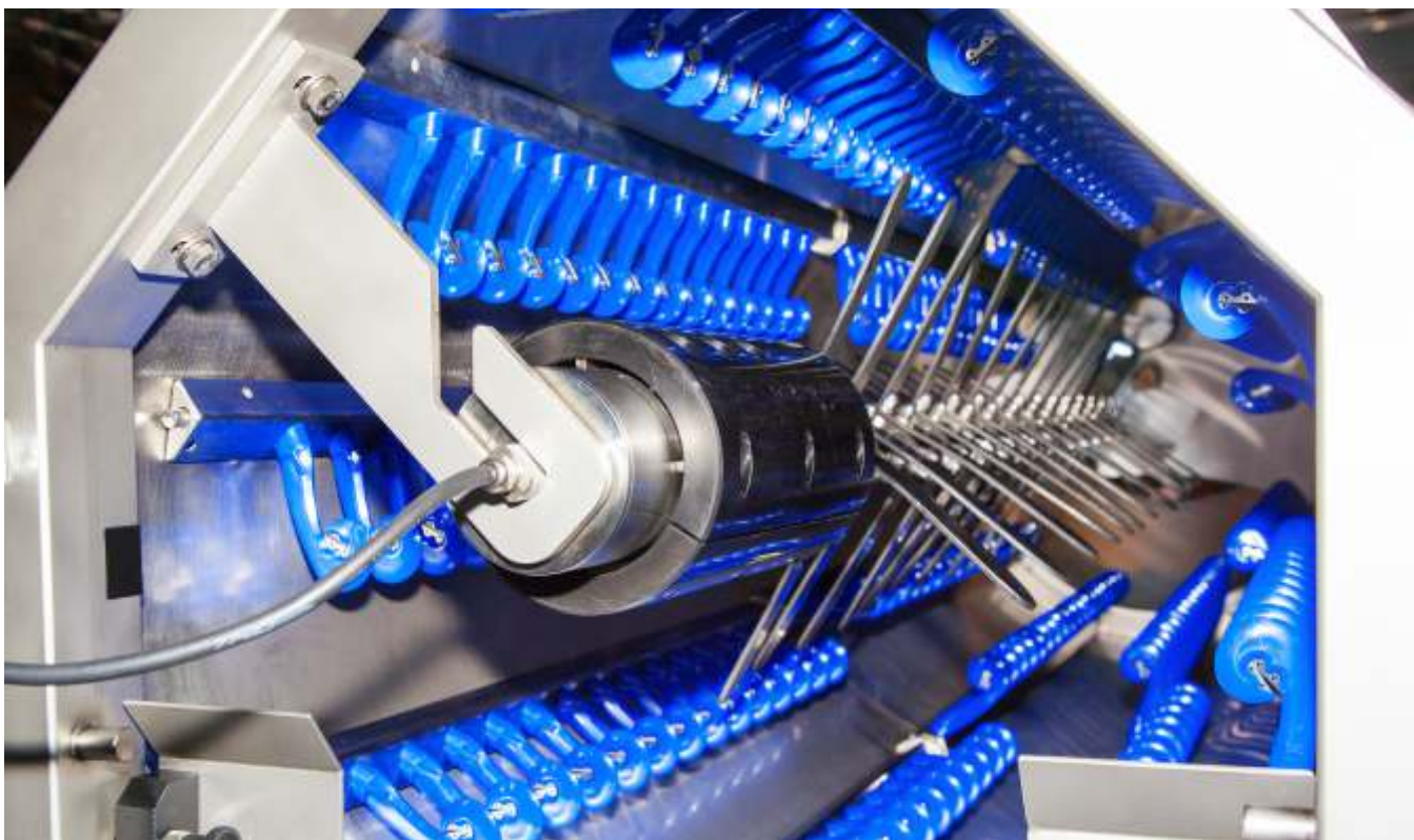
PT 87 X (RVS) als aandrijving van een roerwerk in de vleesindustrie
