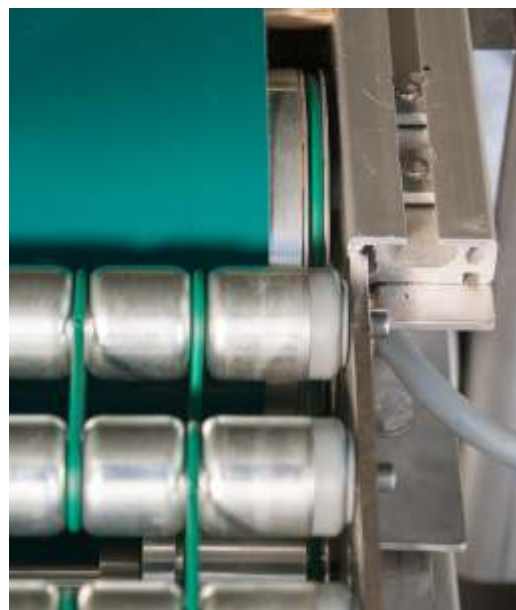
PT 113 X2 met speciaal deksel met daarin een 5 mm brede groef voor een rondsnaar (zie foto rechts), die een korte rollenbaan mee aandrijft
