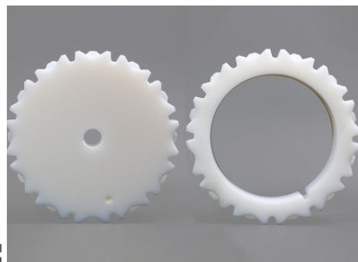
Kettingwiel kunststof - origineel en uitgedraaid
