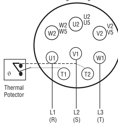
High voltage - Y
